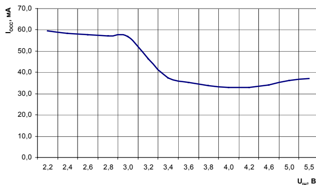
Рисунок 17 Зависимость динамического тока потребления от входного напряжения высокого уровня, при: U_{сс}=5,5 \text{ В} , U_{иL}=0,8 \text{ В} , f=40 \text{ МГц} , T=25^{\circ}\text{C}
