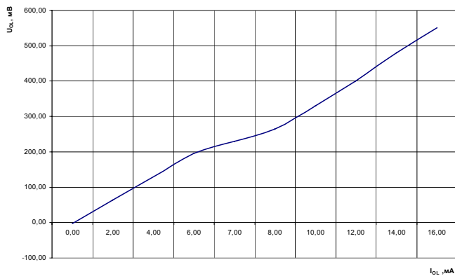
Рисунок 12 Зависимость выходного напряжения низкого уровня от тока нагрузки, при T=25^{\circ}\text{C}
