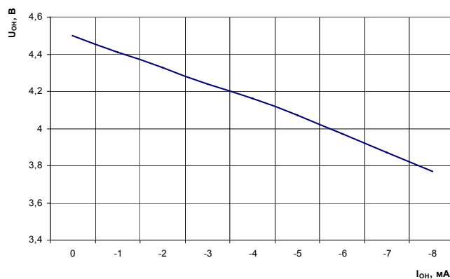
Рисунок 13 Зависимость выходного напряжения высокого уровня от тока нагрузки, при T=25^{\circ}\text{C}
