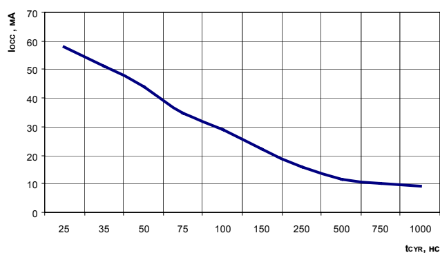
Рисунок 15 Зависимость динамического тока потребления от времени цикла считывания информации t_{CYR} при U_{CC}=5,5 \text{ В} и T=25^{\circ}\text{C}
