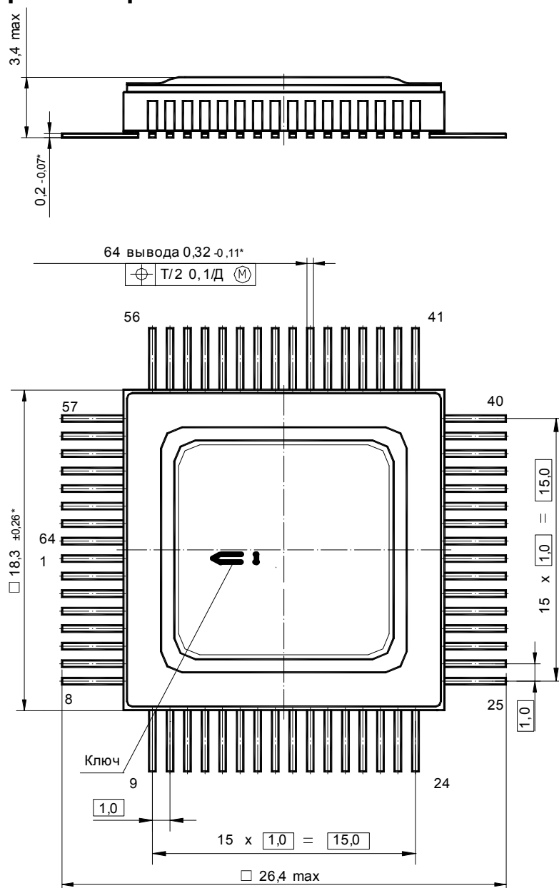
Рисунок 29 Корпус 5134.64-6
