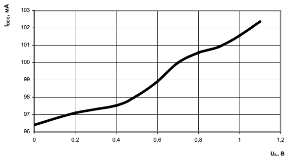
Рисунок 24 Зависимость динамического тока потребления от входного напряжения низкого уровня, при: U_{CC0} = 3,6 В, U_{CC} = 1,98 В, U_{IH} = 2,0 В, f = 33 МГц, T = 25 °С
