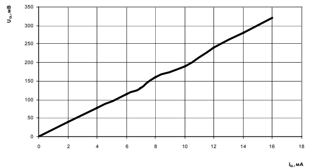
Рисунок 17 Зависимость выходного напряжения низкого уровня от тока нагрузки при U_{CC0} = 3,0 В, U_{CC} = 1,62 В, T = 25 °С
