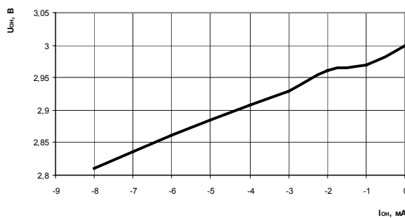
Рисунок 18 Зависимость выходного напряжения высокого уровня от тока нагрузки при U_{CC0} = 3,0 В, U_{CC} = 1,62 В, T = 25 °С
