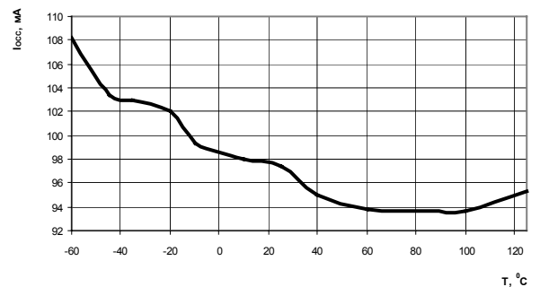
Рисунок 19 Зависимость динамического тока потребления от температуры при U_{CC0} = 3,6 В, U_{CC} = 1,98 В, t_{CYR} = 25 нс
