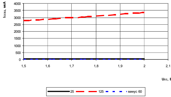
Рисунок 14 Зависимость тока потребления в режиме хранения, КМОП уровни на входах, от напряжения питания матрицы при U_{CC0} = 3,6 В
