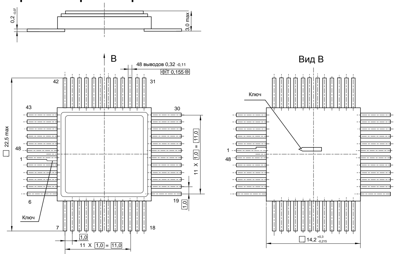
Рис.28 Габаритный чертеж микросхемы в корпусе N16.48-1B
