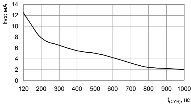
Рис.24 Зависимость динамического тока потребления от времени цикла считывания информации t_{CYR} при: U_{CC}= 3,3 \text{ В} , T=25 \text{ }^\circ\text{C}
