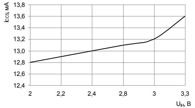
Рис.19 Зависимость тока потребления в режиме хранения, от входного напряжения высокого уровня при: U CC =3,3 В, U IL =0,8 В, f= 25 МГц, T=25 °С
