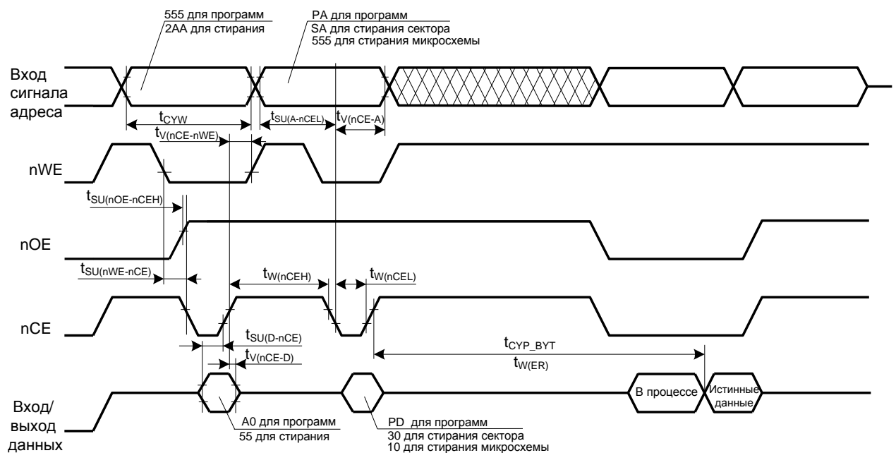
Рис.13 Временная диаграмма цикла записи 1. Управление по nWE. U nOE =U ИН на протяжении цикла записи
