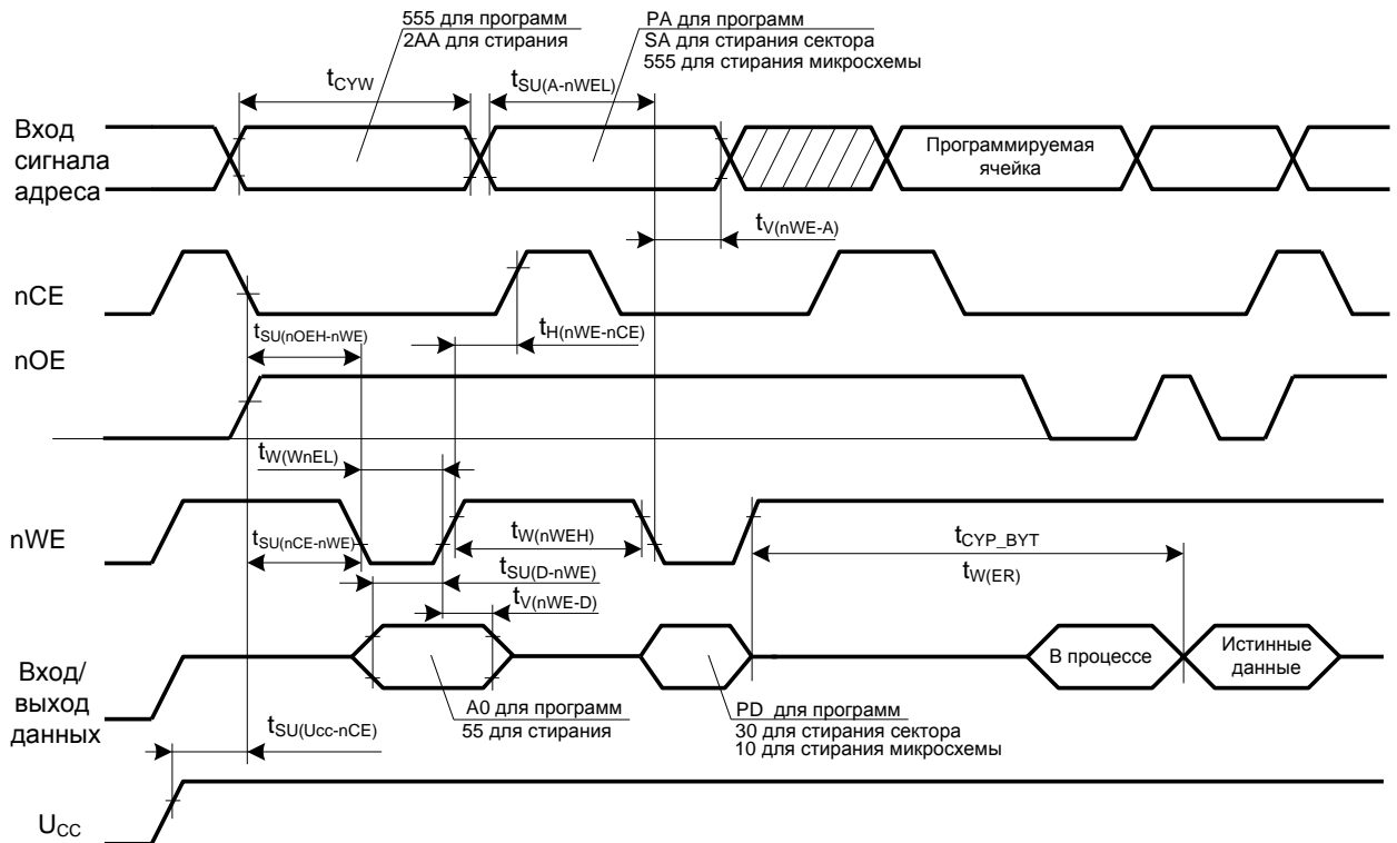
Рис.13 Временная диаграмма цикла записи 1. Управление по nWE. U nOE =U ИН на протяжении цикла записи
