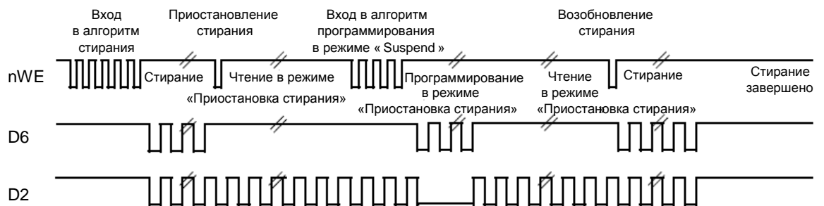
Рис.16 Временная диаграмма переключения статусных бит. Система может использовать nCE или nOE для переключения D2 и D6. D2 переключается только при чтении по адресу внутри стираемого сектора
