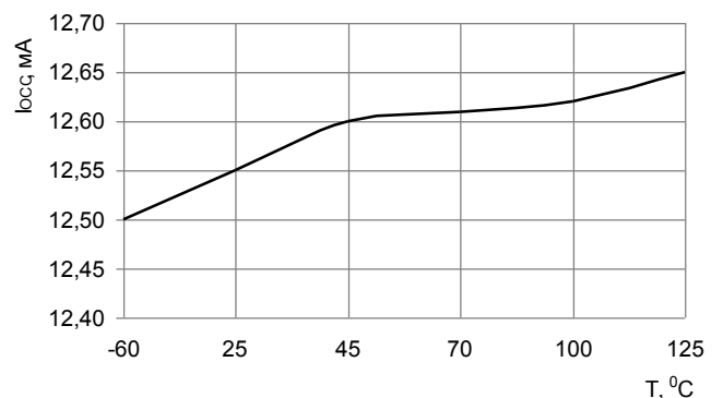
Рис.23 Зависимость динамического тока потребления от температуры при: U CC = 3,3 В, t CYR =120 нс
