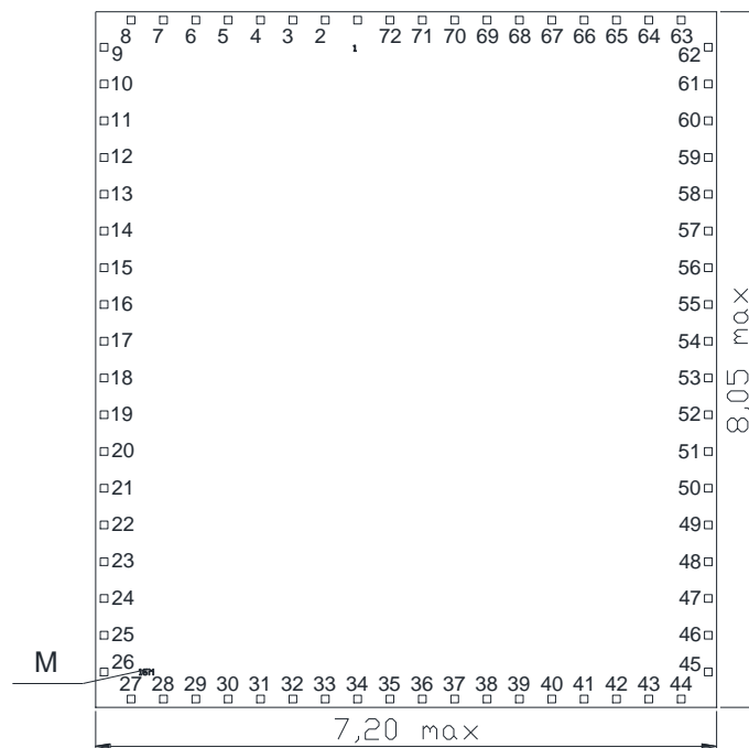
Рис.29 Кристалл (бескорпусное исполнение)
