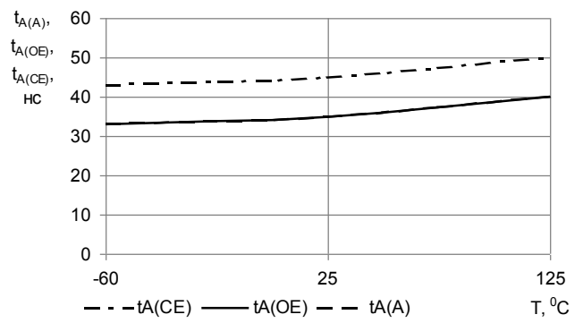
Рис.27 Зависимость времени выборки адреса, t_{A(A)} , времени выборки по сигналу nCE , t_{A(nCE)} , времени выборки по сигналу nOE , t_{A(nOE)} , от температуры при U_{CC}= 3,0 \text{ В}
