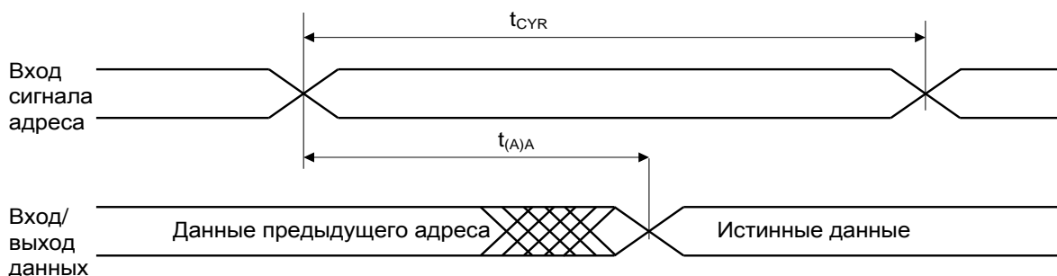
Рис.11 Временная диаграмма цикла чтения 1. U_{nOE} = U_{nCE} = U_{IL}, U_{nWE} = U_{IH}
