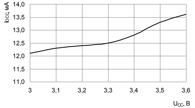
Рис.25 Зависимость динамического тока потребления от напряжения питания при T= \text{минус } 60 \text{ }^\circ\text{C}
