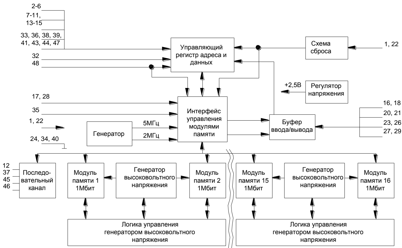
Рис.1 Структурная блок-схема
