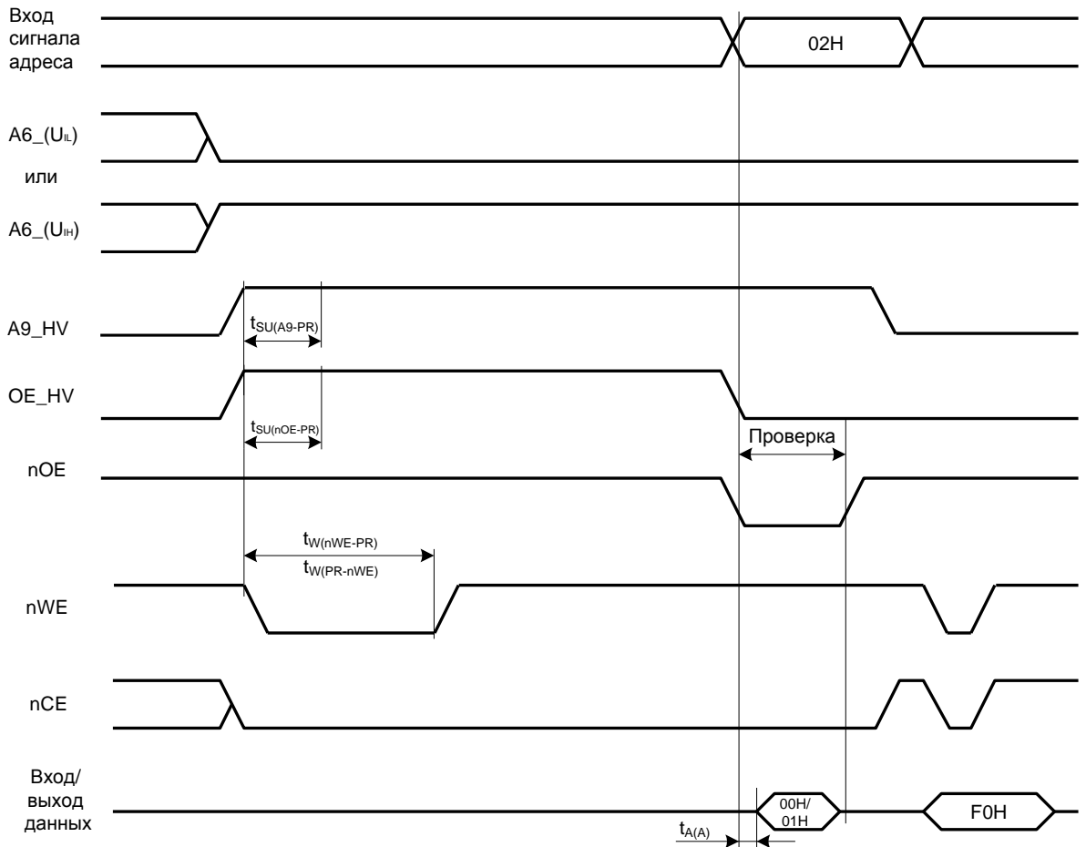
Рис.15 Временная диаграмма цикла защиты/снятия защиты
