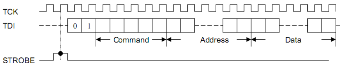
Рис.7 Режим командного цикла
