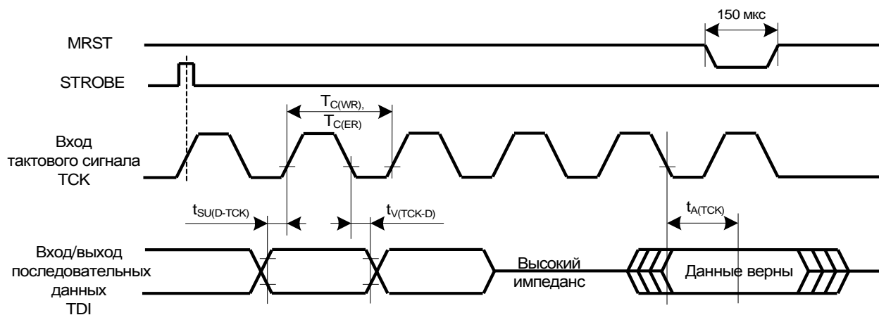
Рис.17 Временная диаграмма записи/чтения последовательного канала STROBE=1 – последовательный канал MRST – параллельный канал
