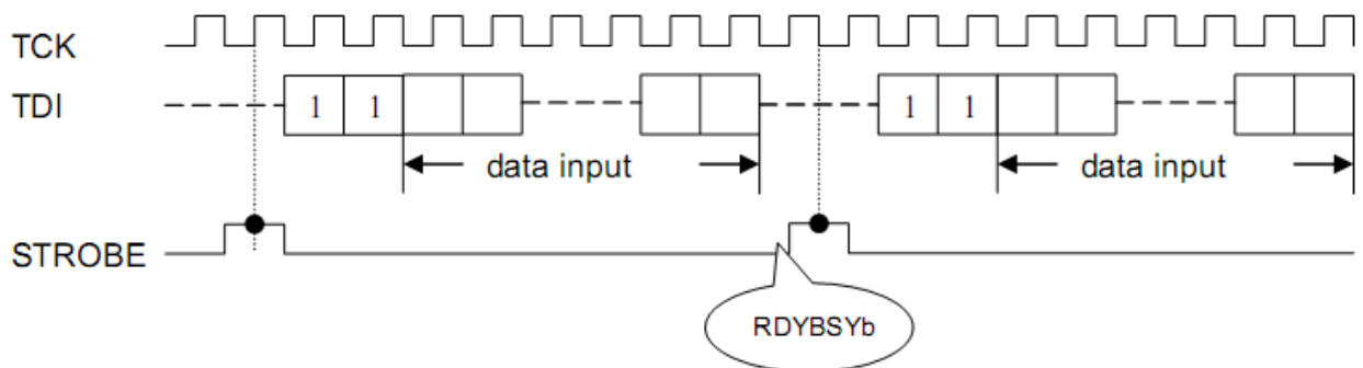
Рис.10 Повтор цикла записи
