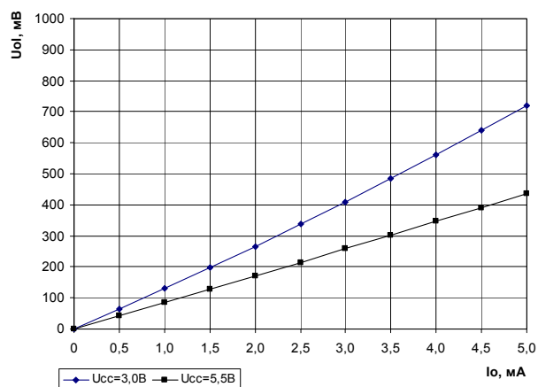
Рис. 6 Зависимость выходного напряжения низкого уровня приемника от напряжения источника питания.
