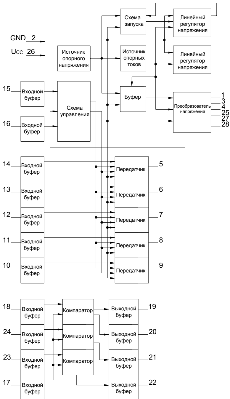
Рис. 1 Структурная блок-схема
