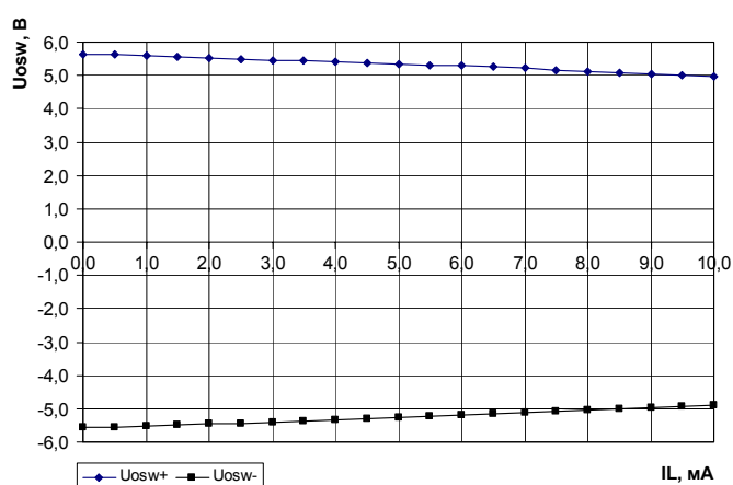
Рис. 12 Зависимость выходного напряжения передатчика от тока нагрузки (нагрузка на выходах 4 передатчиков 3 кОм.).
