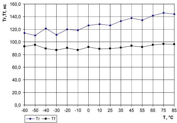
Рис. 21 Зависимость времени нарастания/спада сигнала от температуры ( U_{CC}=4,5 В, C_H=1000 пФ, R_H=3 кОм, режим МВАUD).
