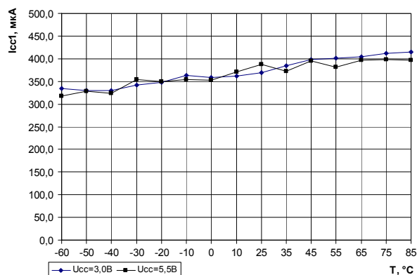
Рис. 4 Зависимость тока потребления в состоянии "Включено" без нагрузки от температуры.
