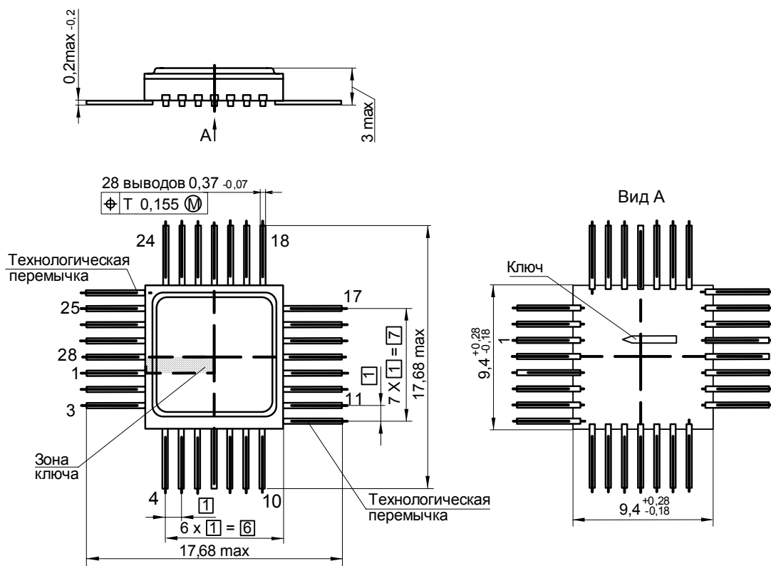
Рис. 23 Корпус H09.28-1B
