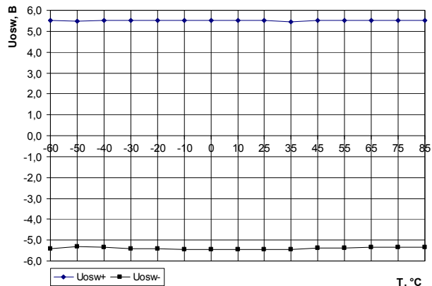
Рис. 14 Зависимость выходного напряжения передатчика от температуры (нагрузка на выходах 5 передатчиков 3 кОм.).
