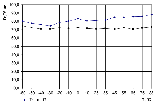
Рис. 18 Зависимость времени нарастания/спада сигнала от температуры (Ucc=3,0 В, CH=1000 пФ, RH=3 кОм).
