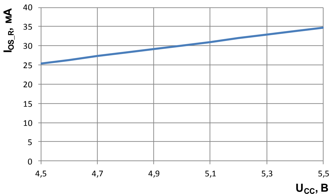
Рисунок 5 – Зависимость тока короткого замыкания выхода приемника I_{OS\_R} от напряжения источника питания при T = 25 °C
