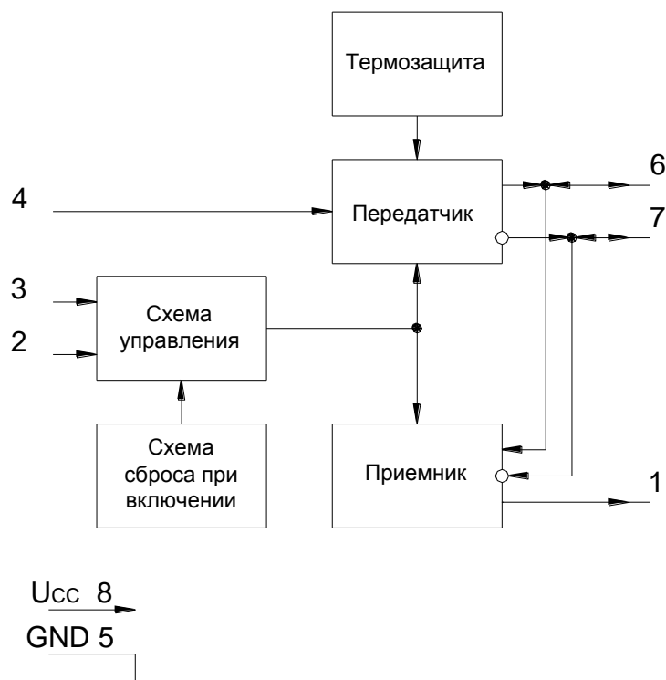
Рисунок 1 – Структурная блок-схема микросхемы
