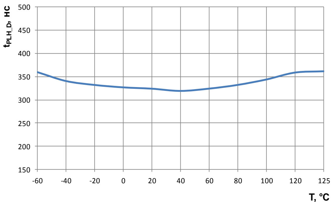
Рисунок 8 – Зависимость времени задержки распространения сигнала передатчика при включении t_{PLH\_D} от температуры при: U_{CC} = 4,5 В
